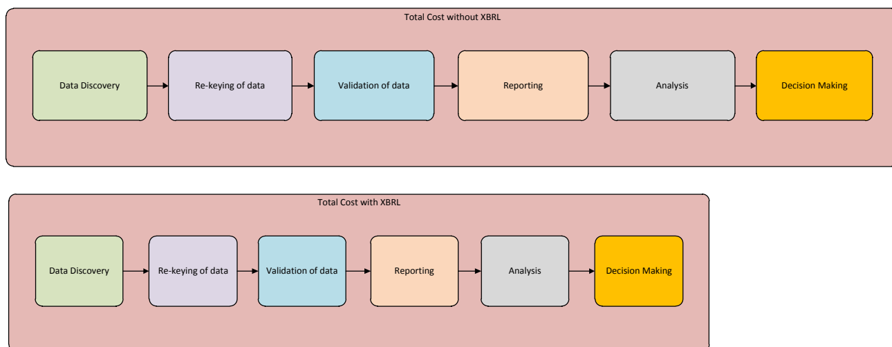
Figura 2. Optimización XBRL
